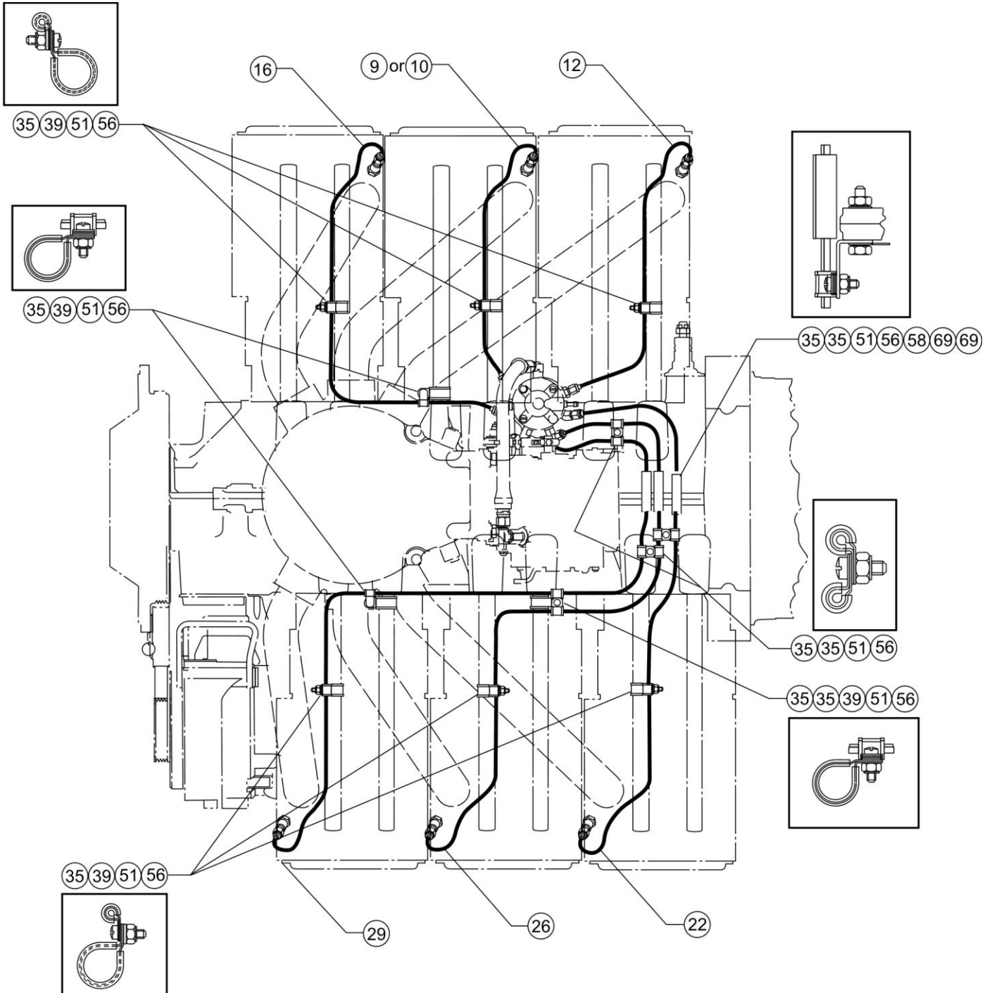
Diagram No. 24 (Optional) -- IO-540-AC1A5 TIO-540-AJ1A
